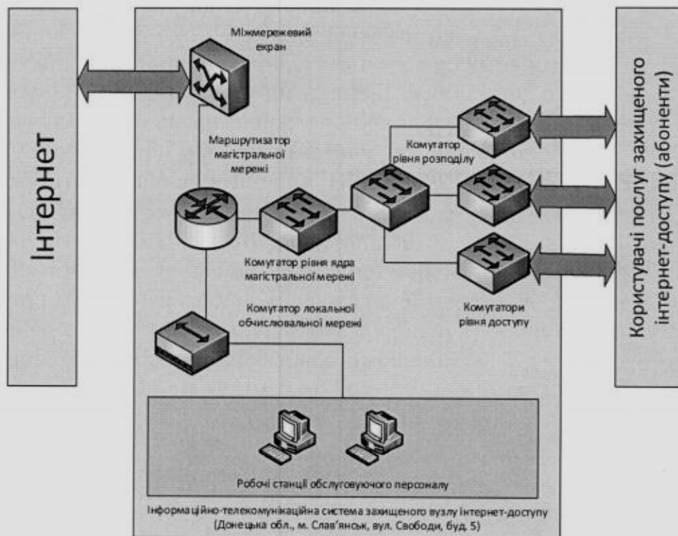
Рис. 2.1. Структурна схема ІТС
